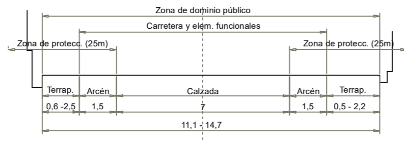
Sección vial CV-50
