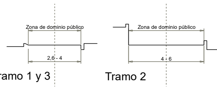
Secciones vial Camí dels Cremats
